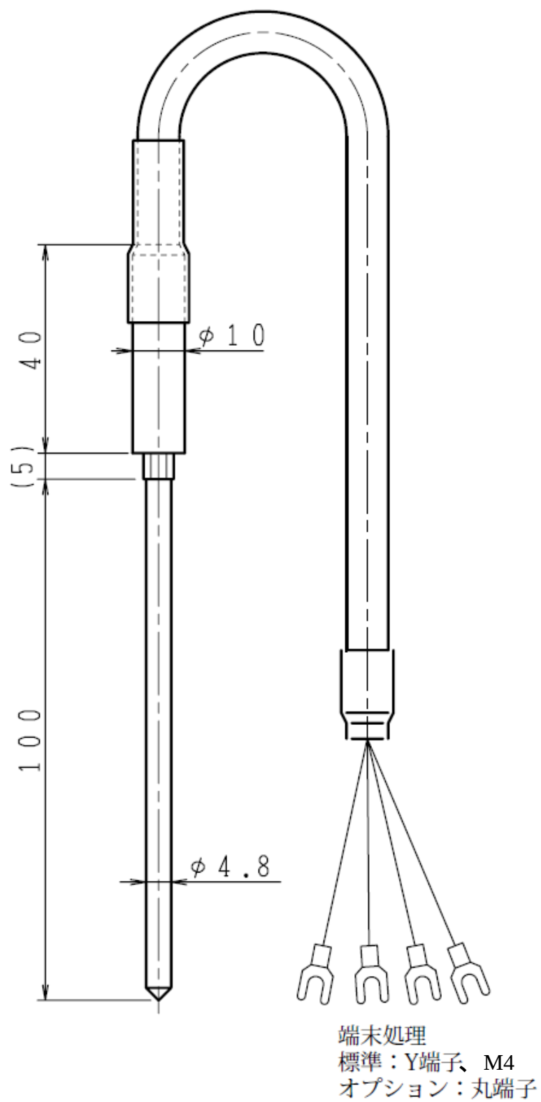
図 3-2 気温測定素子寸法図
