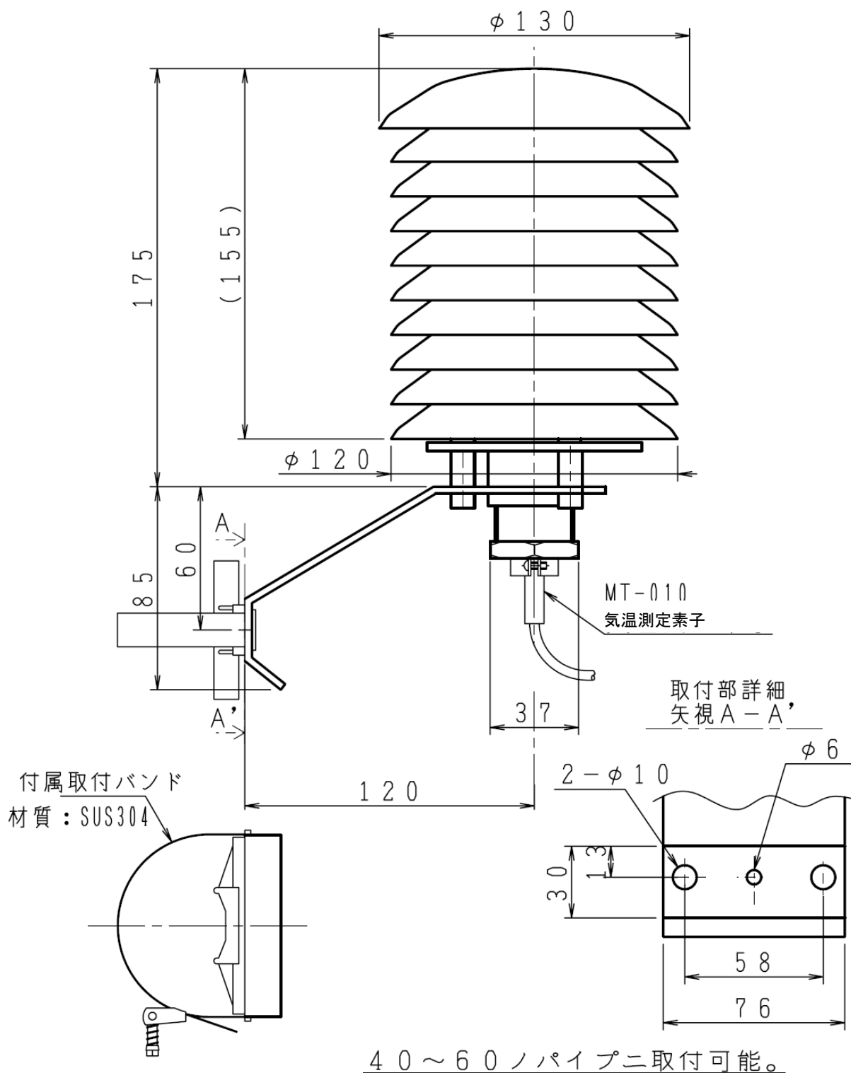
図 3-1. ラジエーションシールド寸法図
