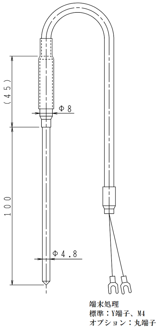
図 3-3. 気温測定素子(MT-010-T)寸法図
